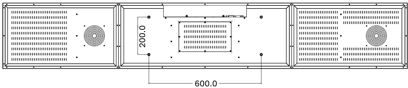
СХЕМА ДИСПЛЕЯ (ВИД СЗАДИ)
